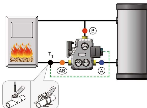
Монтаж вдясно от котела.
