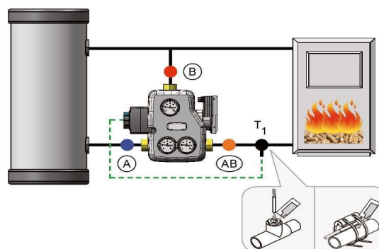
Монтаж вляво от котела.
