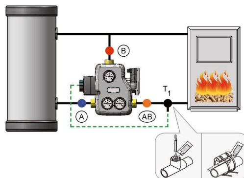
Монтаж вляво от котела.
