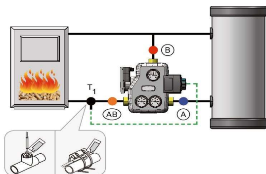
Монтаж вдясно от котела.
